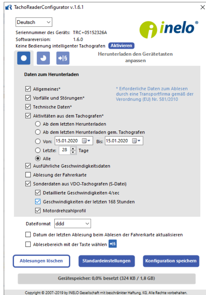
Abb. Konfigurationsfenster: TachoReader Combo Plus.
