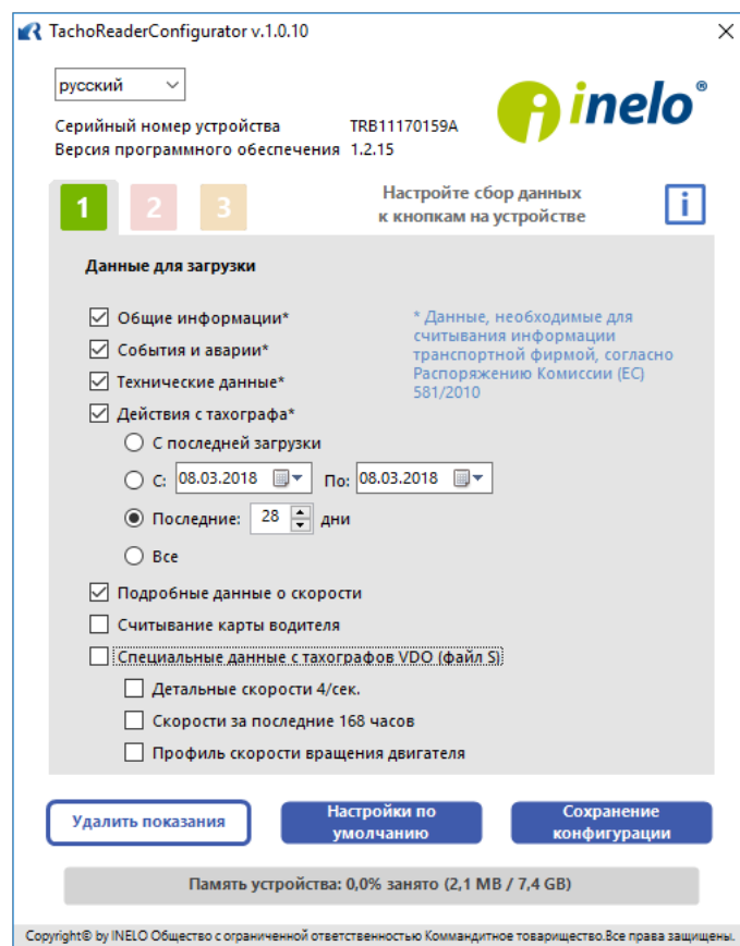
Мал. Вікно конфігурації приладу.
